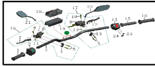
方向把总成 HANDLEBAR ASSY. SECTION 3
