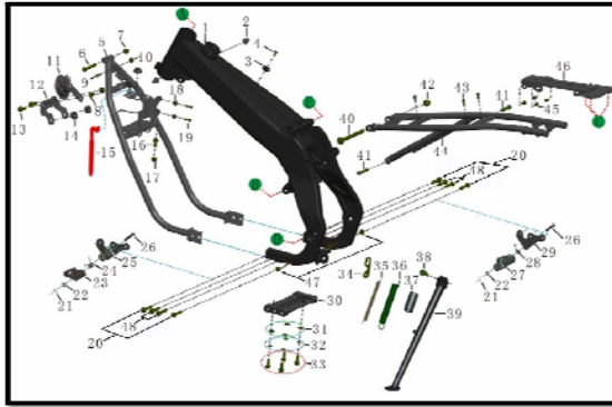
车架和车尾架总成 FRAME AND SUB-FRAME . SECTION 8
