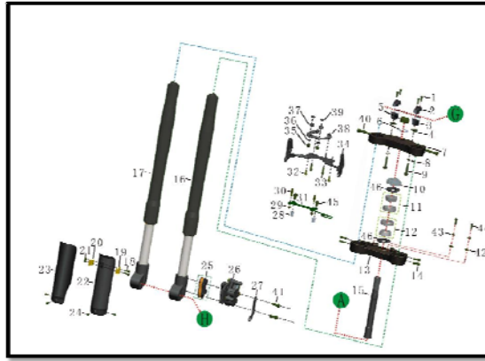
前叉总成 FORK ASSY., FRONT . SECTION 4
